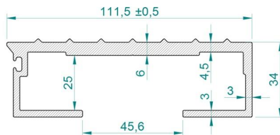
031-008-004 4014 LÁMINA PISO MÓVIL 21 STD CARGO e=6 mm AL6082 T6 (2,668 Kg/m)
