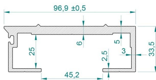
031-008-019 4385 LÁMINA PISO MÓVIL 24 L AL6082 T6 (2,287 Kg/m)
