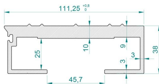
031-008-019 4385 LÁMINA PISO MÓVIL 24 L AL6082 T6 (2,287 Kg/m)
