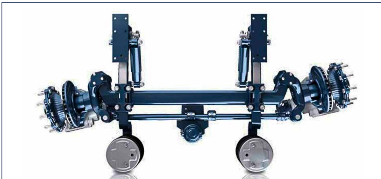
MONTAGE DU TROISIÈME ESSIEU AUTODIRECTIONNEL BPW AVEC RUPTURE
