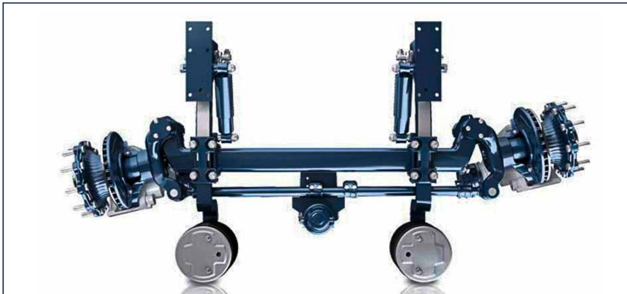
MONTAJE DE 3ER EJE AUTODIRECCIONAL BPW CON QUIEBRO
